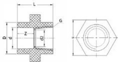
Муфта переходная для раструбной сварки с ВР РР-Н IPS d32 PN10
