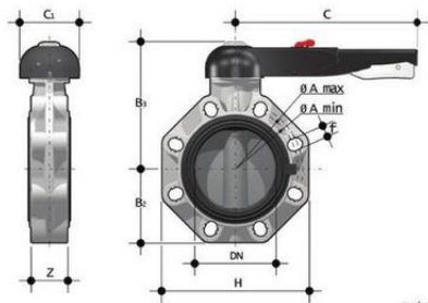
Дисковый затвор промышленного применения FKOMLM с рукояткой (уплотнение FKM) PP-H d160
