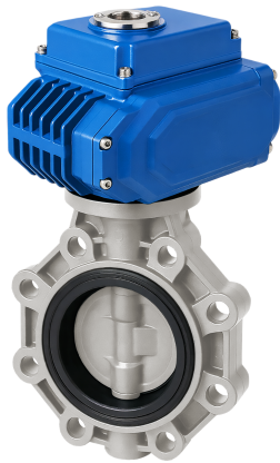
Дисковый затвор IFK PP-H с электрическим приводом 24V DC, EPDM, IPS d225 (DN200)
