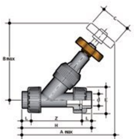
Угловой вентиль VVUIV PBX с разборными муфтовыми окончаниями, EPDM, FIP d50 (DN40)
