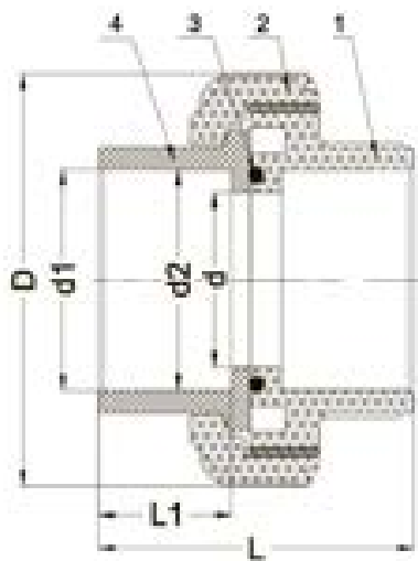
Муфта разборная для раструбной сварки PP-H IPS (FKM) d75 PN10
