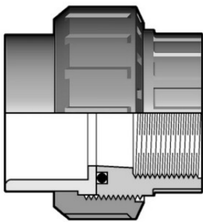
Муфта разборная с ВР ПВХ FIP 75x2½"
