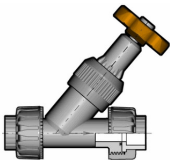
Угловой вентиль VVUIV PBX с разборными муфтовыми окончаниями, EPDM, FIP d40 (DN32)
