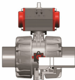
Шаровой кран VKD ПВХ с пневмоприводом НЗ с втулочными окончаниями, FKM, FIP d90 (DN80)
