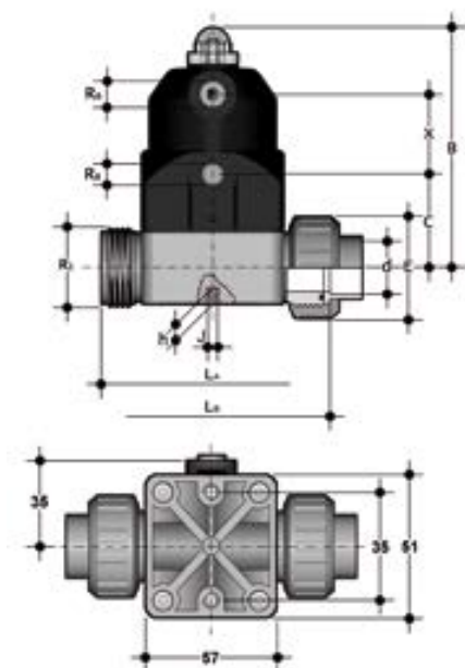
Компактный мембранный клапан CM ХПВХ с пневмоприводом ДвД, втулочные окончания d20 (DN15)
