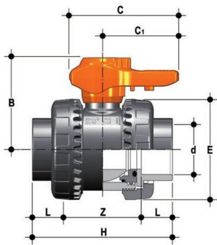
Шаровой кран общего применения VXE ХПВХ с муфтовыми окончаниями d50 (DN40)
