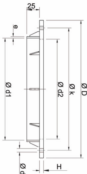
Фланцевый адаптер PPs d90
