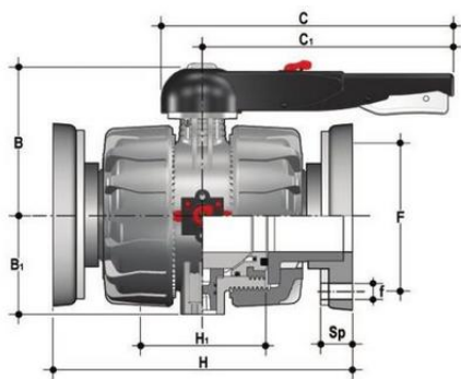
Шаровой кран VKD ПВДФ с фланцевыми окончаниями, DN65-100 d75 (DN65)
