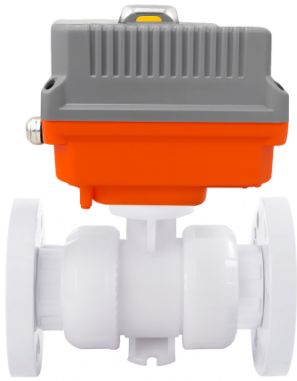
Шаровой кран IVKD ПВХ с эл.приводом 24V DC, фланцевые окончания, EPDM, IPS d20 (DN15)
