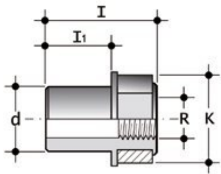
Адаптер с внутренней резьбой PP-H FIP 20x1/2 SDR11 PN6
