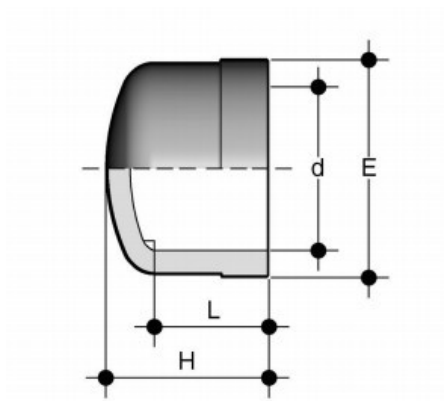
Заглушка клеевая ПВХ FIP d110
