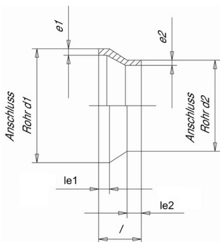
Муфта редукционная PP-H Simona (PN6) 315x280 SDR17.6 PN6
