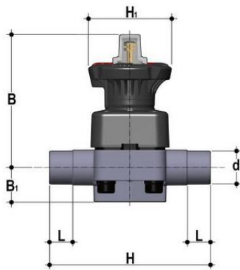
Мембранный клапан DK/L с втулочными окончаниями (уплотнение FKM / мембрана PTFE) PP-H d50 (DN40)
