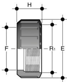
Накидная гайка для BIV ПВХ FIP 1/2
