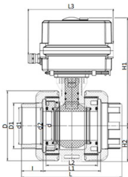
Шаровой кран IVKD ПВХ с эл.приводом 220V AC, муфтовые окончания, EPDM, IPS d75 (DN65)
