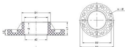
Жесткий фланец ХПВХ IPS (Model B) d225 PN16
