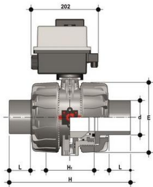
Шаровой кран VKD ПВХ с эл.приводом 24V AC/DC, резьбовые окончания, FKM, FIP d90 (DN80)
