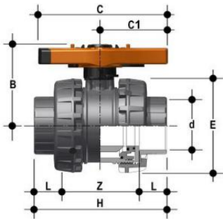
Шаровой кран общего применения VXE ХПВХ с муфтовыми окончаниями, DN65-100 d75 (DN65)
