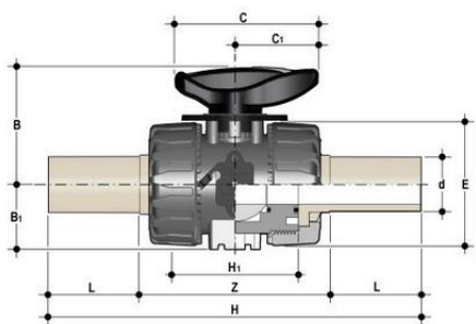
Шаровой кран для регулирования потока VKR с патрубками (CVDM) (уплотнение EPDM) PP-H d32 (DN25)
