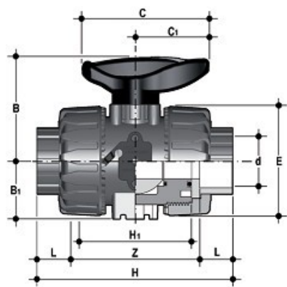
Шаровой кран ПВХ промышленного применения VKD с муфтовыми окончаниями, EPDM, FIP d110 (DN100)
