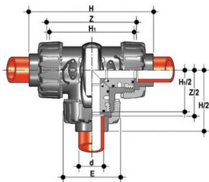
3-х ходовой шаровой кран TKD с муфтовыми окончаниями Т-шар (уплотнение EPDM) PP-H d63 (DN50)
