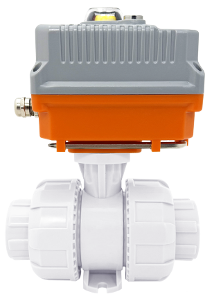
Шаровой кран IVKD ПВДФ с эл.приводом 220V AC, муфтовые окончания, EPDM, IPS d110 (DN100)
