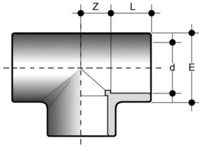
Тройник равнопроходной клеевой 90° ПВХ FIP d225
