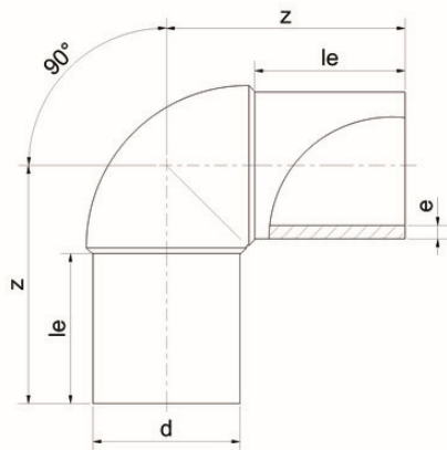
Отвод 90° PP-H Simona d125 SDR11 PN6
