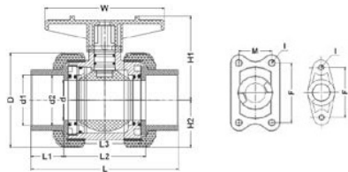
Шаровой кран IVKD ПВДФ с муфтовыми окончаниями d20 (DN15)
