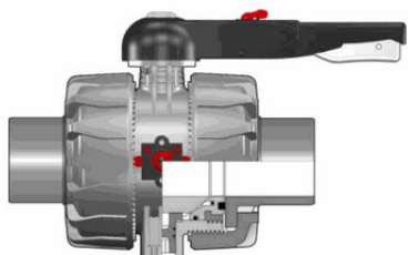
Шаровой кран промышленного применения VKD С втулочными окончаниями (уплотнение FKM) PP-H d90 (DN80)
