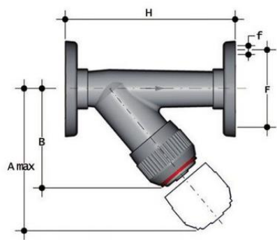
Грязевый фильтр RVOT ПВХ с фланцевыми окончаниями, EPDM, FIP d110 (DN100)
