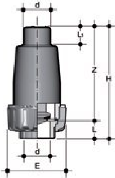
Донный клапан VZIV ПВХ с муфтовыми окончаниями, EPDM, FIP d63 (DN50)
