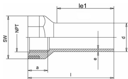
Адаптер переходной с внутренней резьбой ПВДФ (Simona) 32x1" SDR21 PN16
