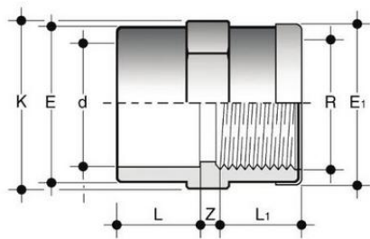
Переходная муфта с усиливающим кольцом ХПВХ 16x3/8" PN16
