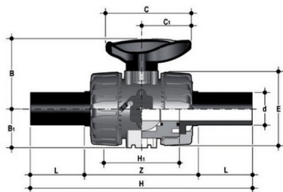
Шаровой кран ПВХ промышленного применения VKD с патрубками из ПЭ (CVDE), EPDM, FIP d50 (DN40)
