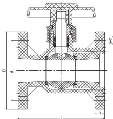
Шаровой кран IVKD ПВДФ с фланцевыми окончаниями d20 (DN15)
