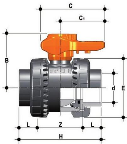
Шаровой кран общего применения VXE ХПВХ с муфтовыми окончаниями d16 (DN10)
