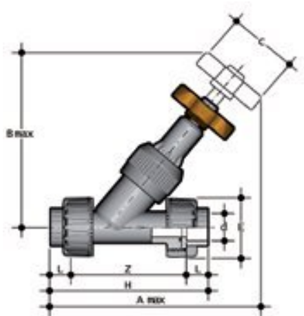
Угловой вентиль VVUIV PBX с разборными муфтовыми окончаниями, EPDM, FIP d32 (DN25)
