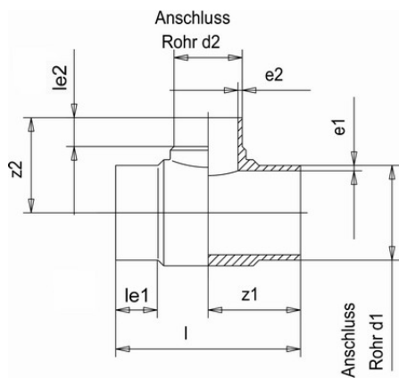
Тройник равнопроходной PP-H Simona (PN6) d110 SDR17.6 PN6
