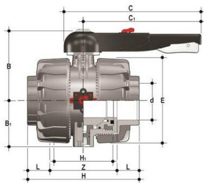
Шаровой кран промышленного применения VKD ХПВХ с муфтовыми окончаниями, DN65-100 d110 (DN90)
