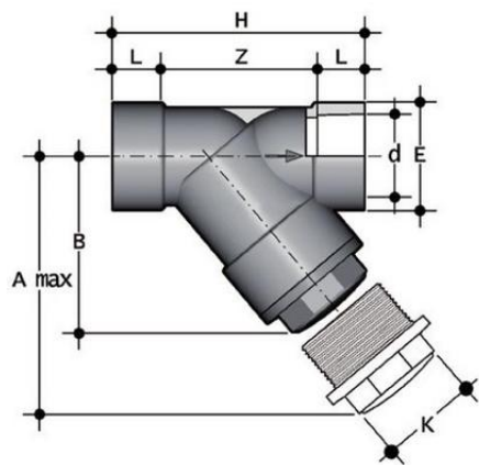
Грязевый фильтр RVIV PBX с муфтовыми окончаниями, EPDM, FIP d110 (DN100)
