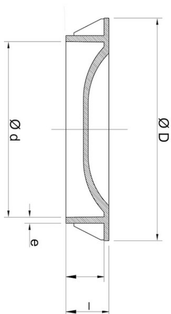
Фланцевая заглушка PPs d125
