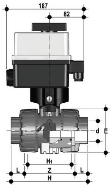
Шаровой кран VKD ПВХ с эл.приводом 90-240V, муфтовые окончания, FKM, FIP d63 (DN50)
