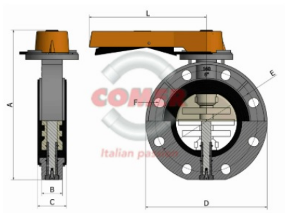
Дисковый затвор ПВХ с рукояткой, EPDM, Comer d160 (DN150)
