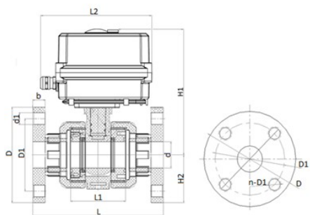
Шаровой кран IVKD ПП-гомополимер с эл.приводом 220V AC, фланцевые окончания, FKM, IPS d20 (DN15)
