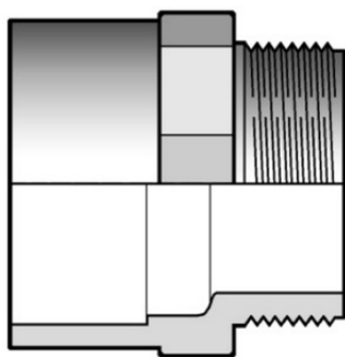
Двойной муфтовый адаптер с НР ПВХ FIP 20x16x1/2
