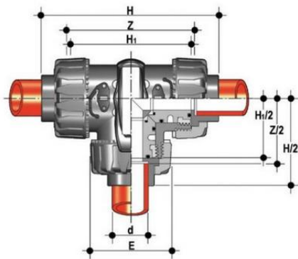
3-х ходовой шаровой кран TKD с муфтовыми окончаниями Т-шар (уплотнение FKM) PP-H d40 (DN32)
