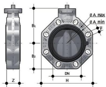
Дисковый затвор ПВХ FKOAVFM со свободным штоком, EPDM, FIP d16" (DN400)
