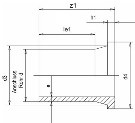
Бурт PP-H Simona d90 SDR11 PN10
