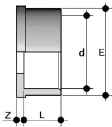
Муфтовое окончание для BIV PBX FIP d16
